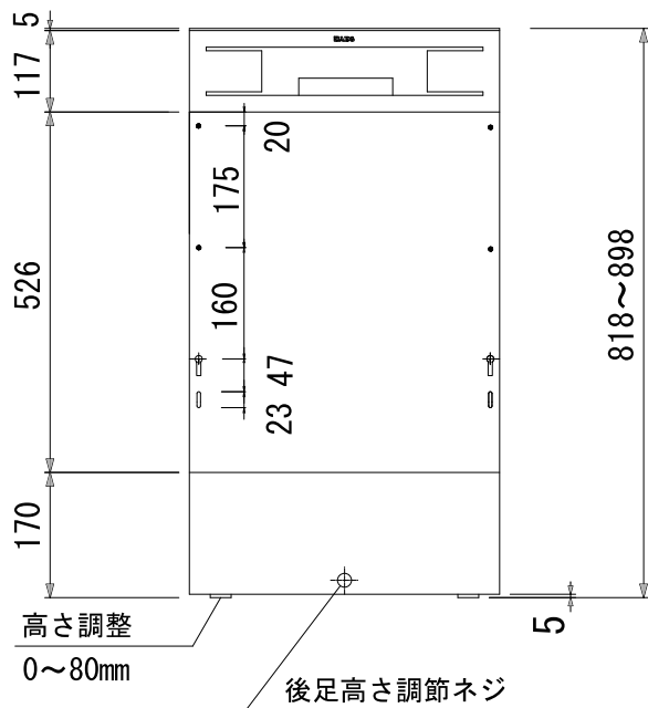
正面図
