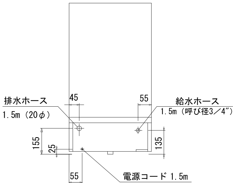
背面図
