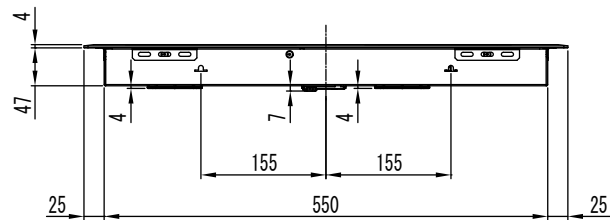
カウンター開口寸法
