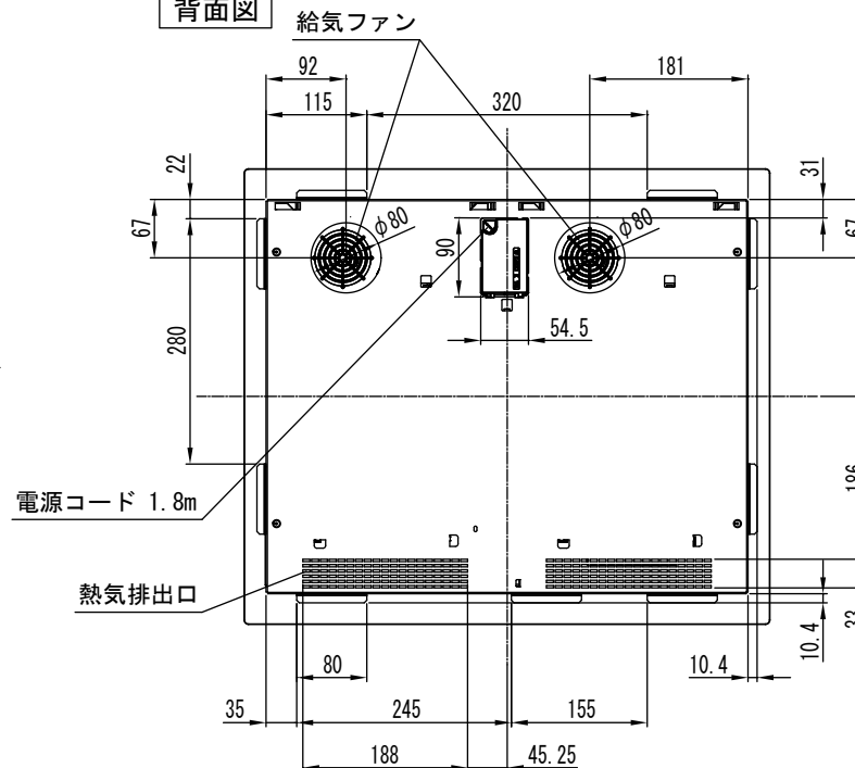
背面図
